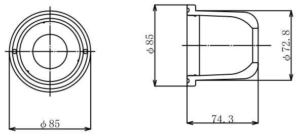
6-1. ベルキャップF (本体) (溶融亜鉛めっき HDZT 77)
