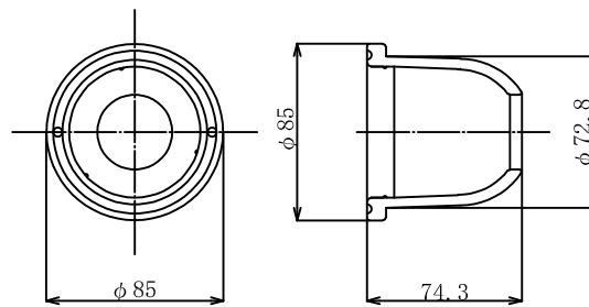
5-1. ベルキャップF (本体) (溶融亜鉛めっき HDZT 77)
