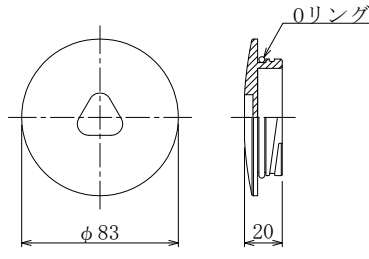
5-2. ベルキャップF (蓋部) (溶融亜鉛めっき HDZT 77)
