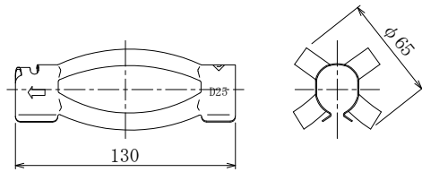
3. K-1スペーサー D25-65 (電気めっき)
