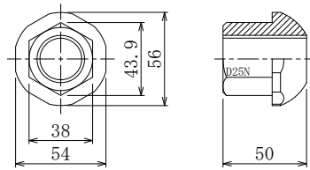
2. ASメッキコマナット D25N (溶融亜鉛めっき HDZT 49)
