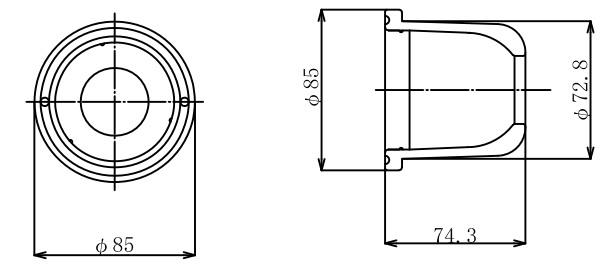
5-1. ベルキャップF (本体) (溶融亜鉛めっき HDZT 77)
