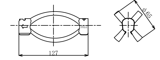
3. K-1スペーサー D22-65 (電気メッキ)
