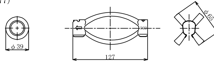
4. K-1スペーサー D22-65 (電気メッキ)
