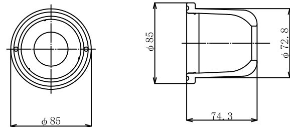
5-1. ベルキャップF (本体) (溶融亜鉛めっき HDZT 77)
