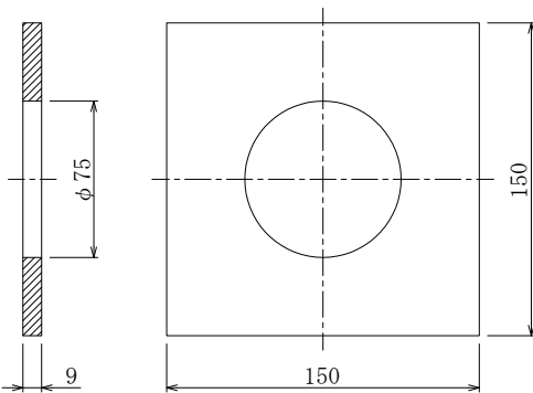
4. メッキ付角座金 (溶融亜鉛めっき HDZT 77)
