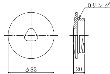
5-2. ベルキャップF (蓋部) (溶融亜鉛めっき HDZT 77)
