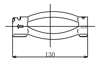
4. K-1スペーサーD25-65 (電気メッキ)
