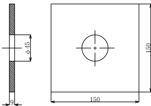
5. 角座金
