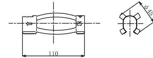
4. K-1スペーサーD25-45 (電気メッキ)
