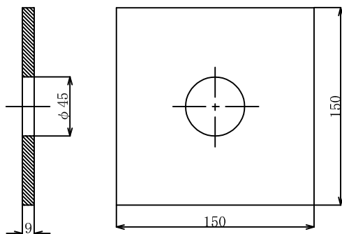
5. 角座金
