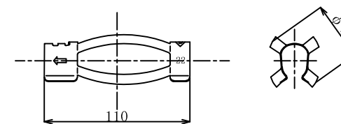
3. K-1スペーサーD22-45 (電気メッキ)
