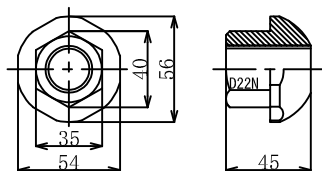
2. ASコマナット D22N
