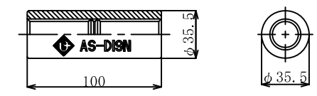
3. AS19カップラー
