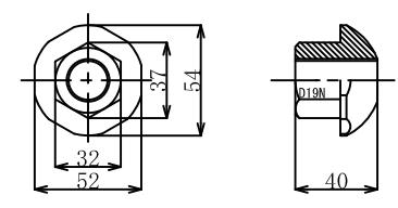
6. 球面ワッシャー
