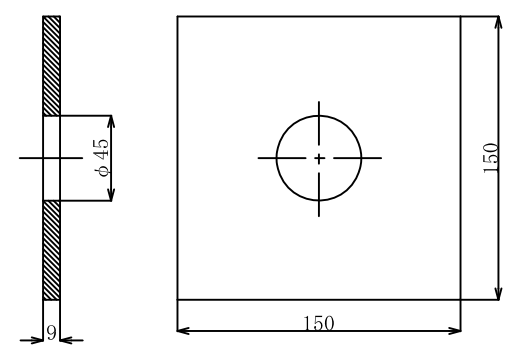
5. 角座金
