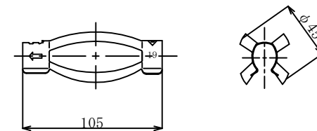
4. K-1スペーサー D19-45 (電気メッキ)
