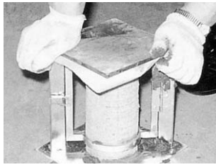
⑤ 整形した供試体の上面をセメントペーストによりキャッピング処理します。(キャッピング用ホルダー使用)
