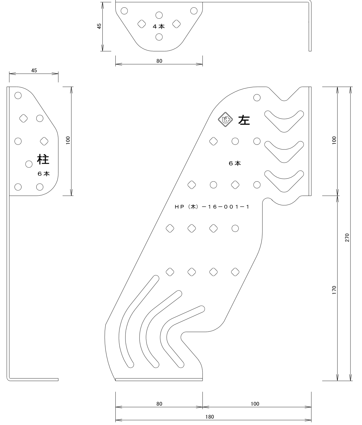
ブレスターZ600 (左)
