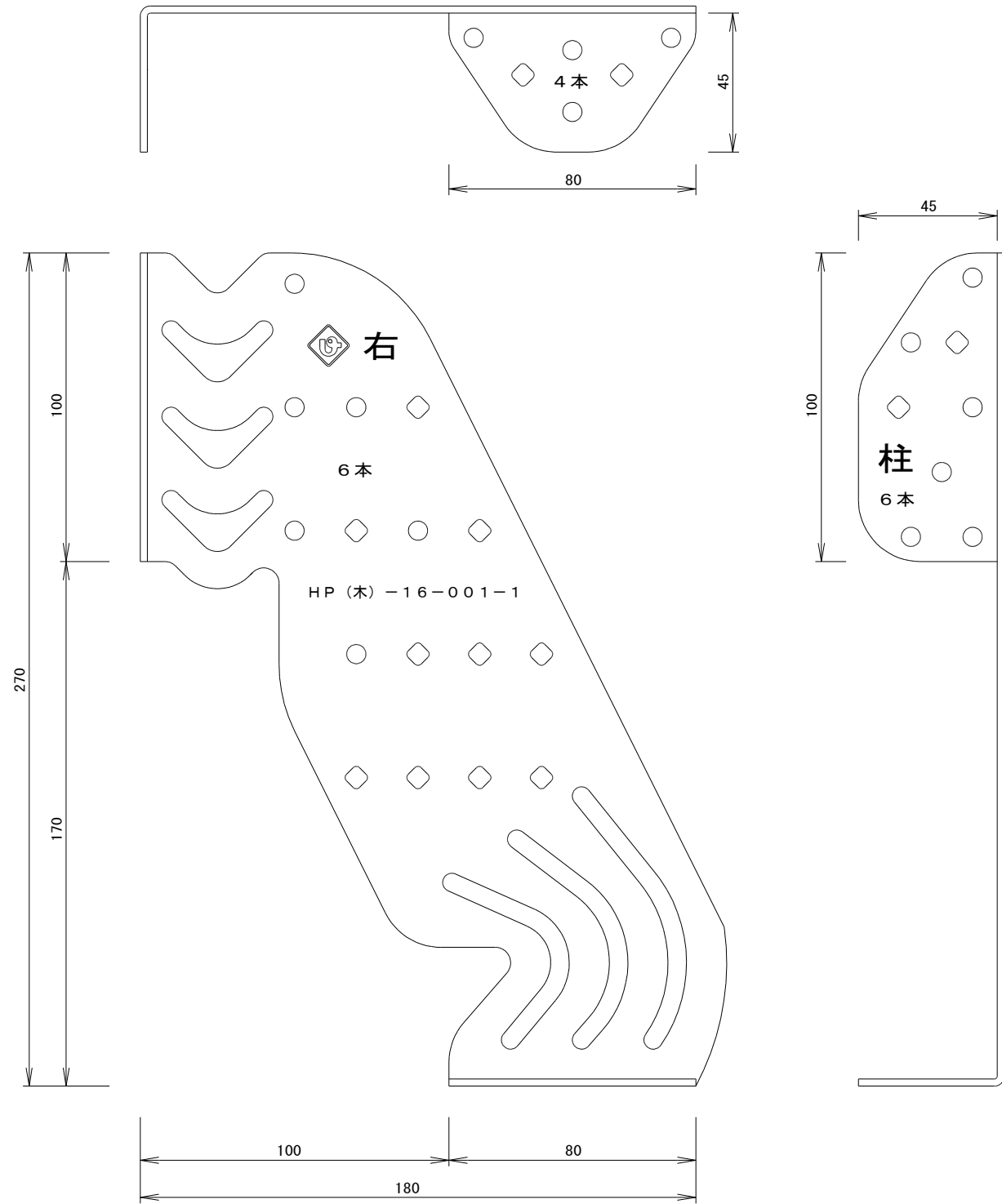
ブレスターZ600 (右)
