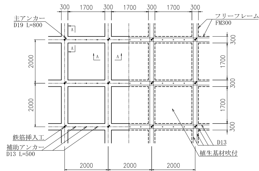
展開図 S=1/100
